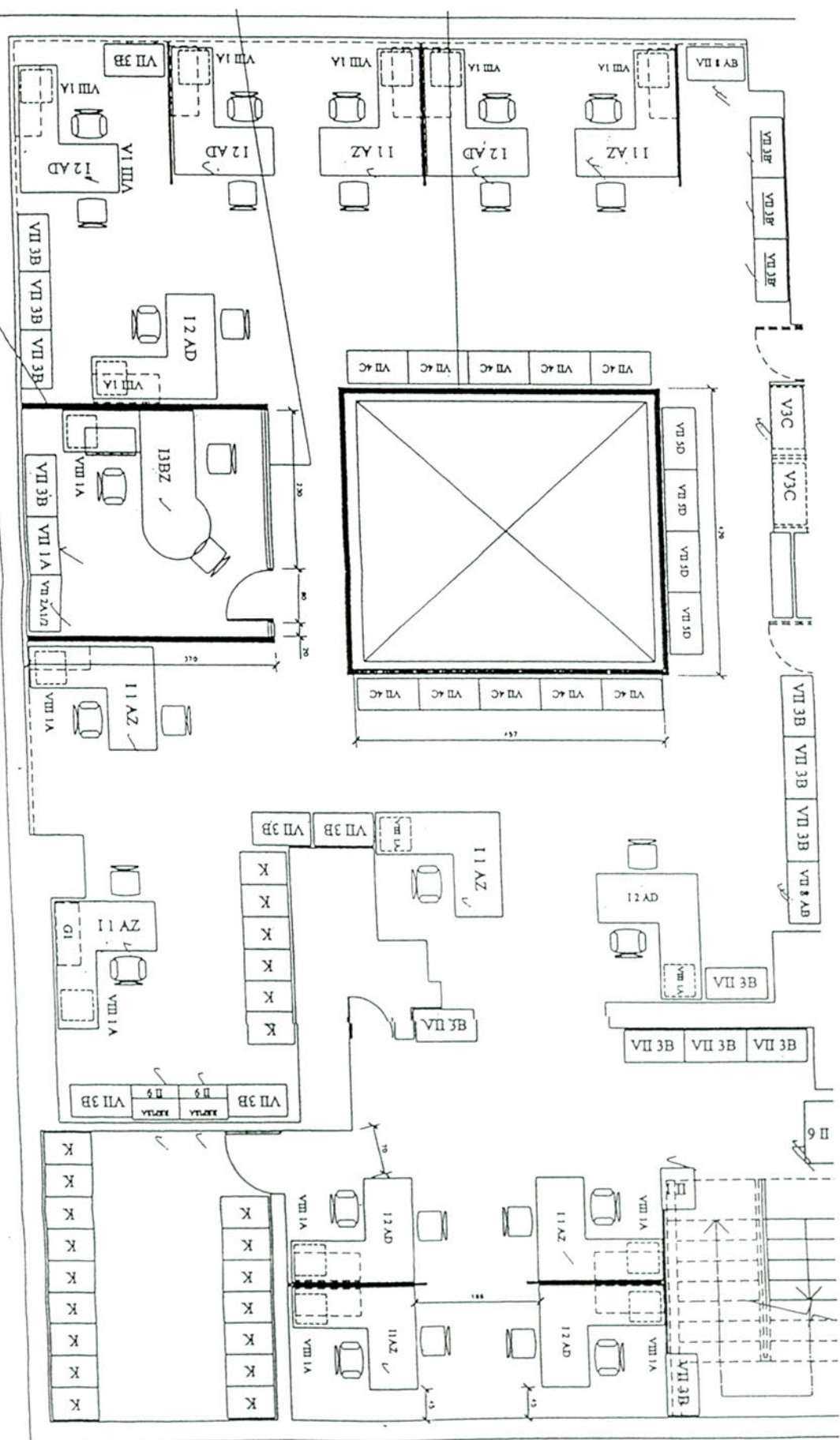
PLANTA ARQUITECTURA ENTREPISO ESCALA 1:50
