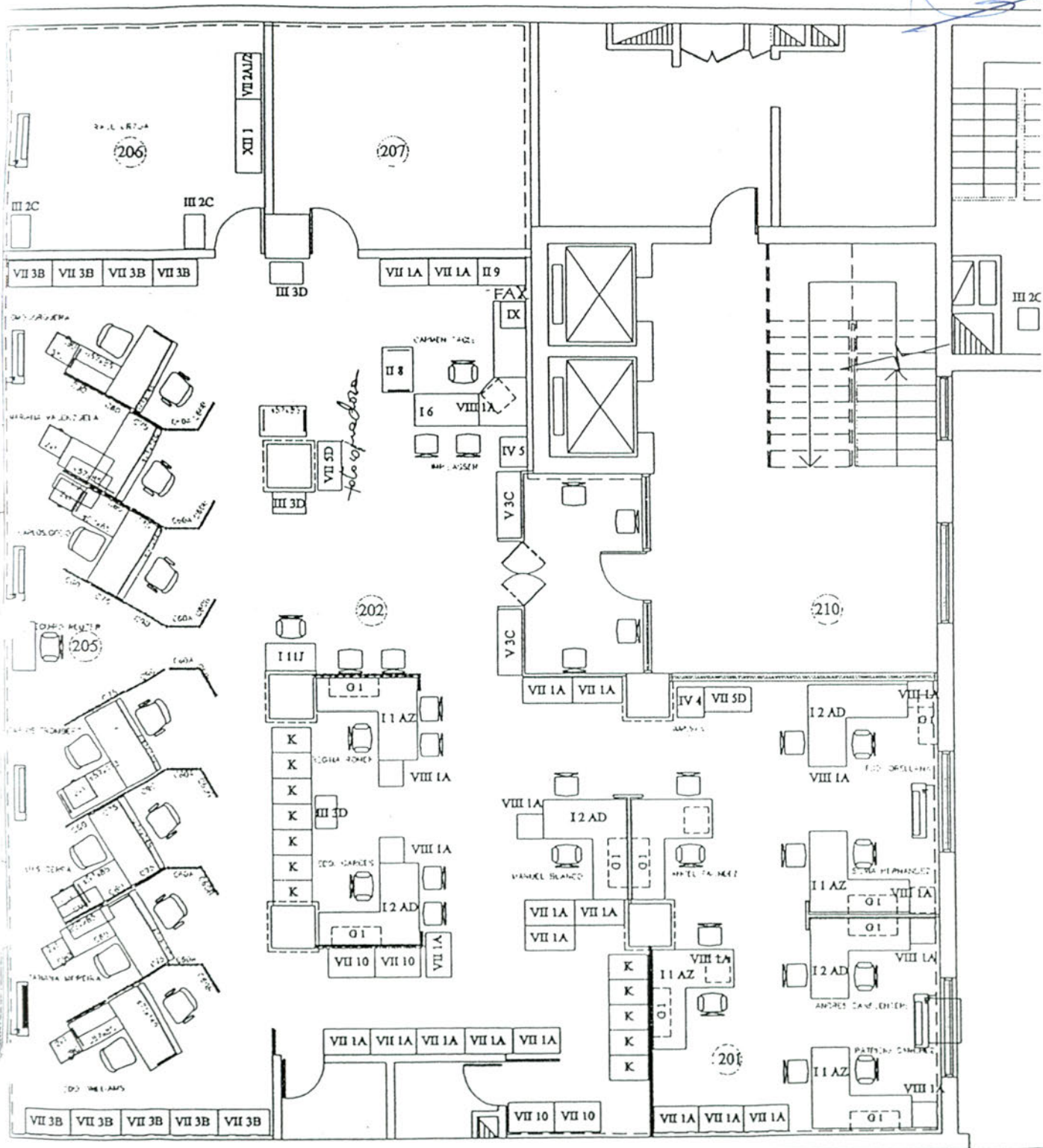
PLANTA ARQUITECTURA 2 PISO ESCALA 1 : 100
